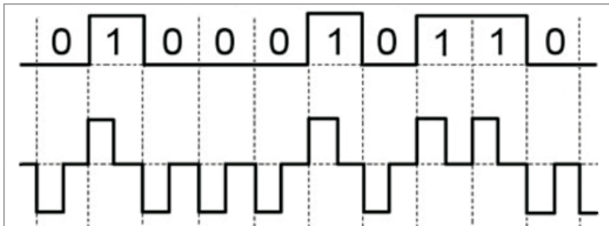
Figura 12: Codifica RZ.
