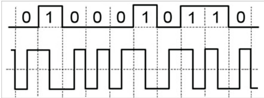
Figura 13: Codifica Manchester.
